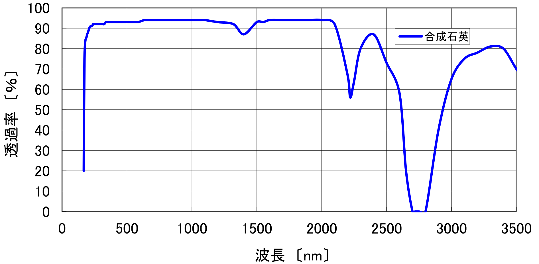
石英透過率波長特性 (T=10mm)
